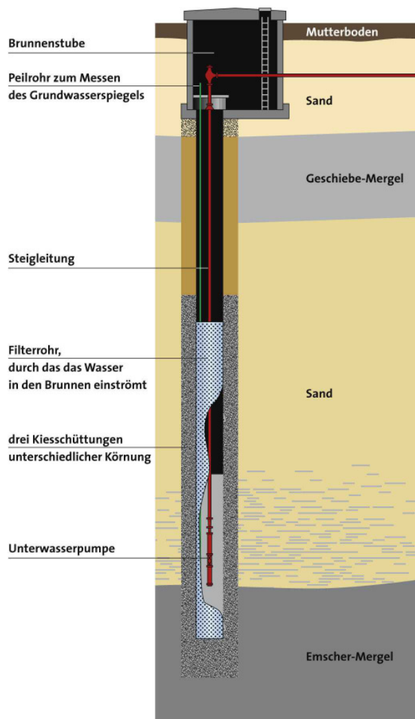
Abb. 20: Aufbau eines Förderbrunnens (Grafik: Stadtwerke Bielefeld GmbH, 2015)
