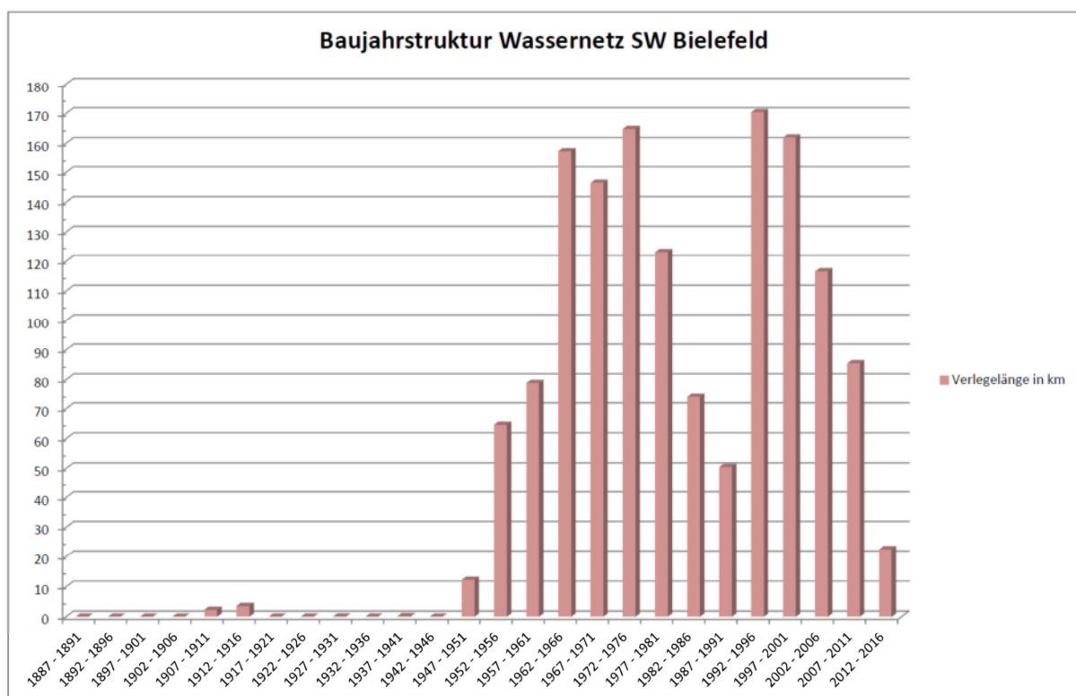
Abb. 31: Baujahrstruktur des Verteilnetzes, (Quelle: Historische technische Jahresberichte der Stadtwerke Bielefeld, Weiterbearbeitung 2017)
