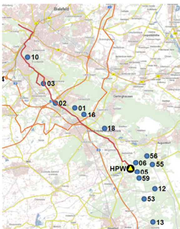
Abb. 27: Lageplan der Zubringerwasserleitung ZW1 mit Darstellung der Wasserwerke (Quelle: Stadtwerke Bielefeld, 2017)
