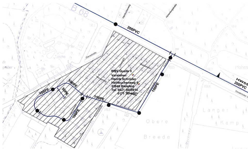
Abb. 21: Lageplan des Wasserbeschaffungsverbandes Quelle II, nicht maßstäbliche Verkleinerung aus dem Geographischen Netzinformationssystem der Stadtwerke Bielefeld, 2017
