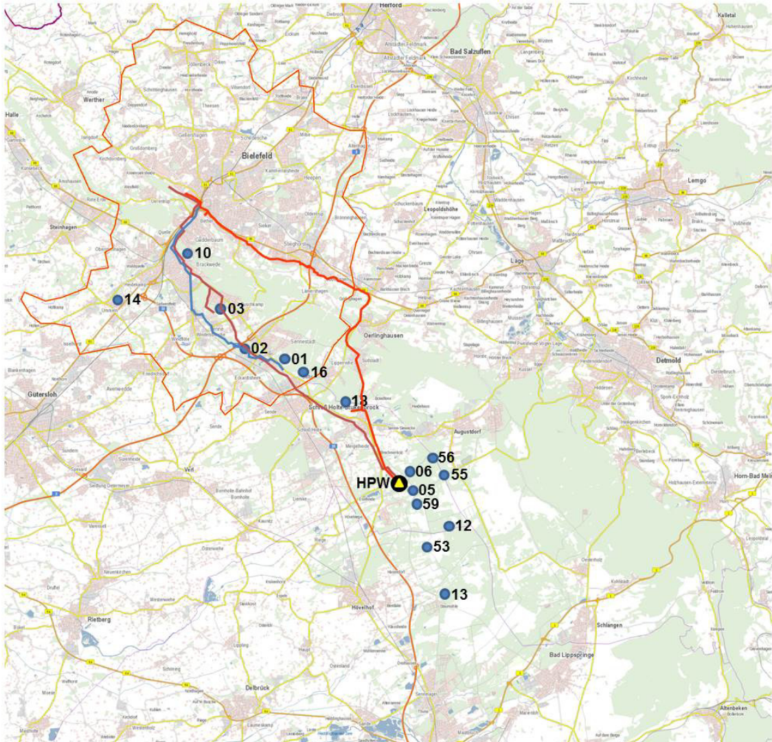
Abb.17: Lageplan Wasserwerke, Zubringerleitungen (ZW), Hauptpumpwerk (HPW)
