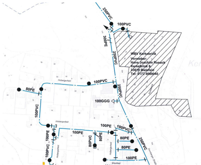
Abb. 23: Lageplan des Wasserbeschaffungsverbandes Kerkebrink, nicht maßstäbliche Verkleinerung aus dem Geographischen Netzinformationssystem der Stadtwerke Bielefeld, 2017
