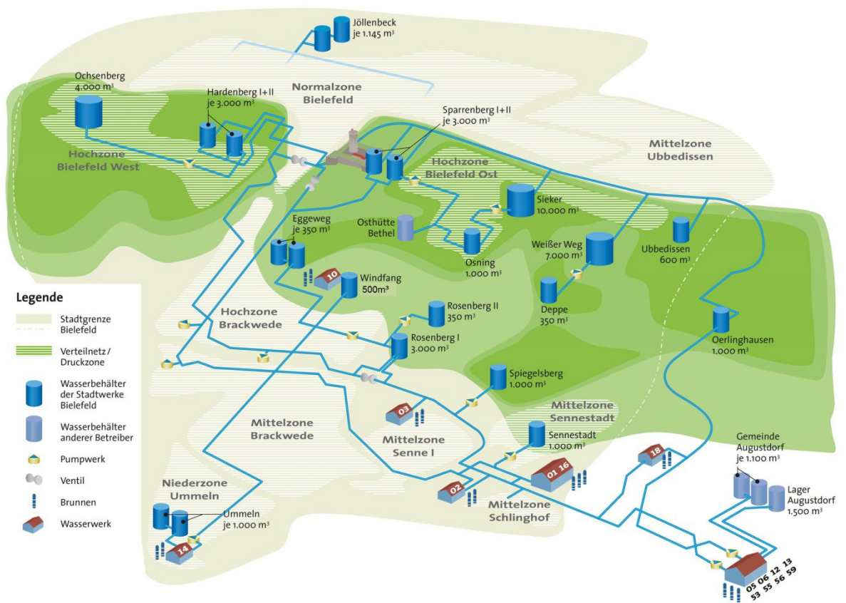
Abb.18: Strukturschaubild Wasserversorgungssystem der Stadtwerke Bielefeld, (Quelle: Stadtwerke Bielefeld, eigene Darstellung 2016, unveröffentlicht)
