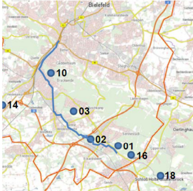
Abb. 29: Lageplan der Zubringerwasserleitung ZW3 mit Darstellung der Wasserwerke (Quelle: Stadtwerke Bielefeld, 2017)
